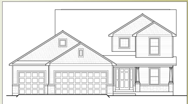
Elevation B
